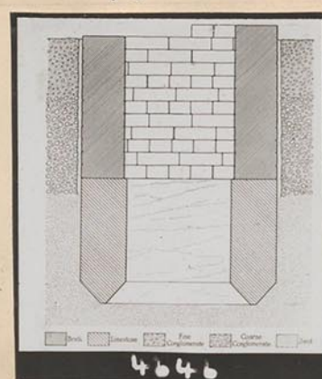
Senkkasten aus Stein, Schnittzeichnung
