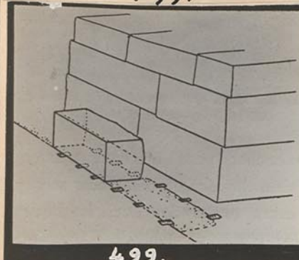
Gîze Granitquader mit Versatzlöchern vor dem Kernmauerwerk.
