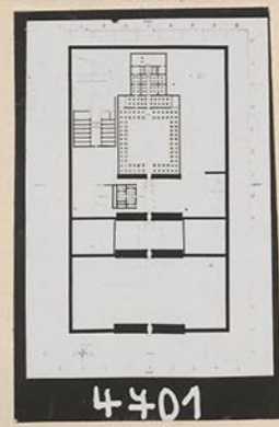
Haremhäb-Befestigung Grundriss n. Hölscher
