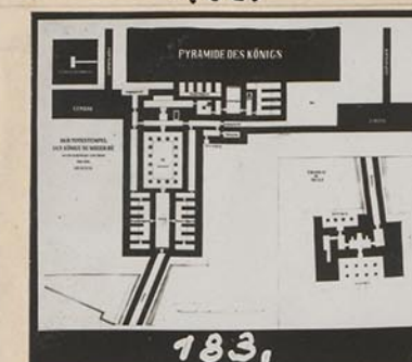
Abuſir Niuserrê, Tempel und Torbau.
