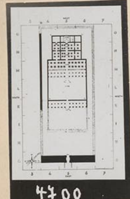
Haremhäb-Befestigung Eje-Bau Grundriss n. Hölscher
