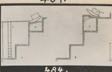
Vorsetzen von Stein- blöcken (Choisy)
