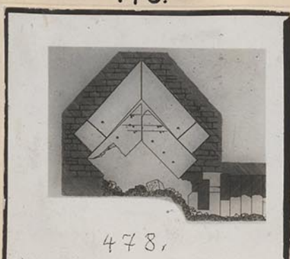
Abusir. Nefertikê. S-N-Schnitt durch die Pyramidenkam- mer.
