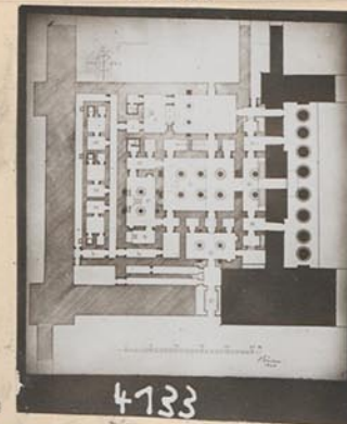
Palast Ramses' III., jüngerer Bau
