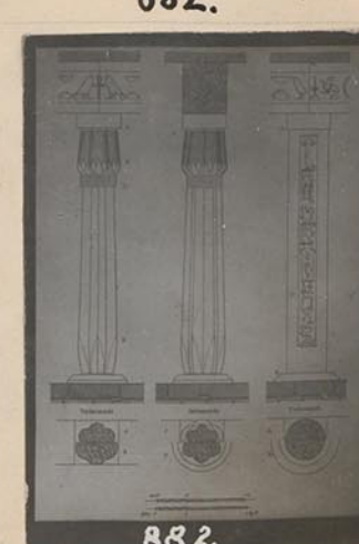
Abusir. Sahurê. Papyrusbündel- und Stamm- säule
