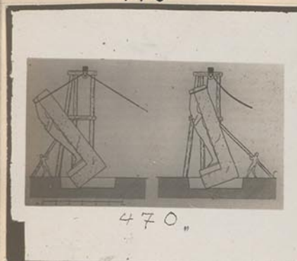
Aufriecher von Kolossalstatuen. (Hölscher)
