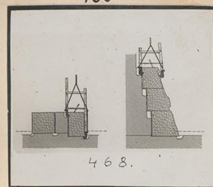
Skizzen des Hebe- raths und Schrauben- vorrichtungen. (Hölscher)
