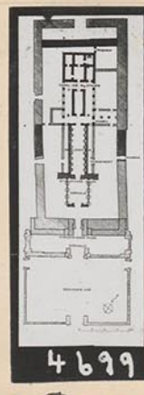
Kleiner Tempel Grundriss n. Hölscher
