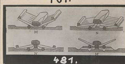
Hebevorrichtung für Steinblöcke (Choisy)
